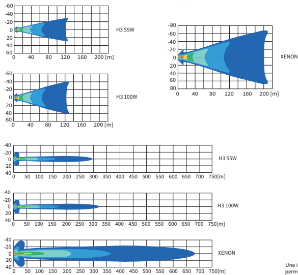
Faisceau lumineux - projection sur la route
